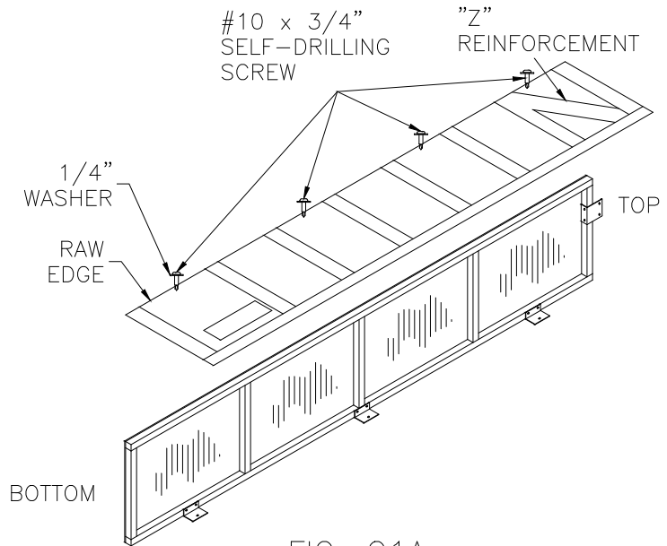
FIG. O1A
