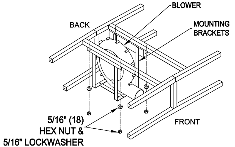
FIG. 13-B
